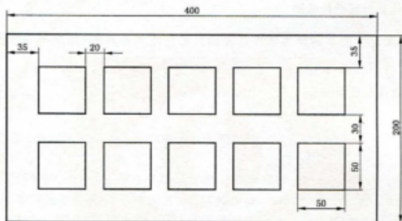
图 1 拉伸粘结强度成型框
